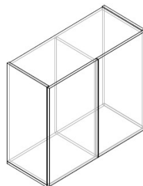
MOBILE MULTIUSO 2A 80 MISURE L 80,9 P 34,8 H 70 CM
