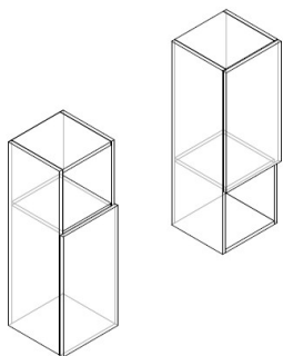
PENSILE VERTICALE MISURE L 30 P 30 H 86,8 CM
