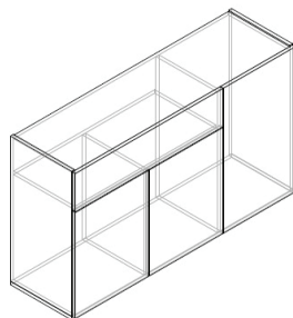
CREDENZA 120 MISURE L 120 P 34,8 H 70 CM
